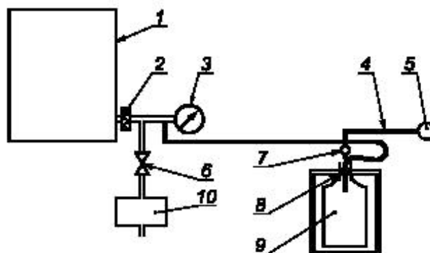
1 — изолирующее устройство; 2 — HEPA-фильтр (опция); 3 — манометр; 4 — резиновая трубка; 5 — пилетка; 6 — изолирующий вентиль; 7 — трубка Парджо; 8 — резиновая пробка; 9 — изолированный стеклянный сосуд; 10 — источник давления или вакуума
